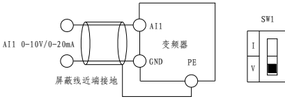
图 2-6 模拟输入端子配线图
