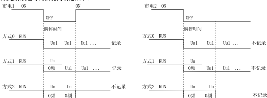
图 5-1-8 瞬停处理
