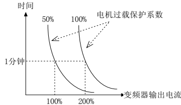
图 5-13-1 电机过载保护系数设定
