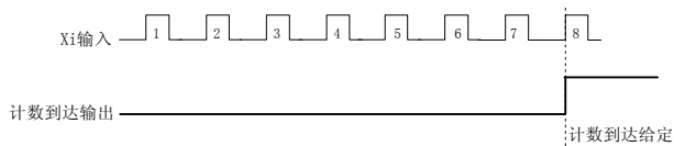
图 5-3-12 计数到达
