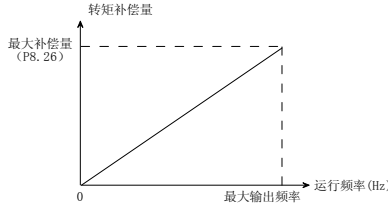
图 5-8-2 高速转矩补偿量与输出频率关系图
