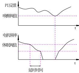
图 5-7-3 休眠和唤醒
