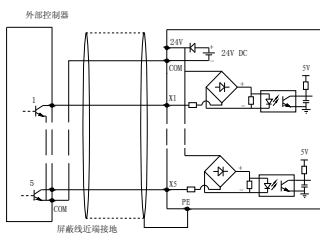
图2-10输入多功能端子配线连接图
