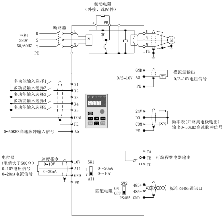
图 2-13 接线图
