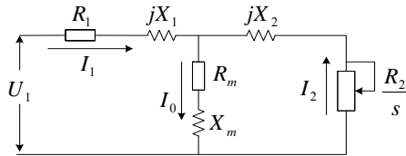
图 5-10-1 异步电机稳态等效电路图
