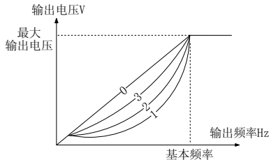
图 5-9-1 降转矩曲线
