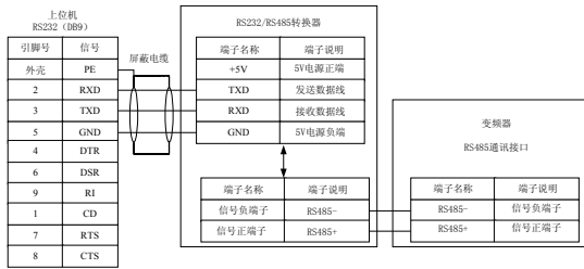
图 2-8 上位机与变频器接口接线图
