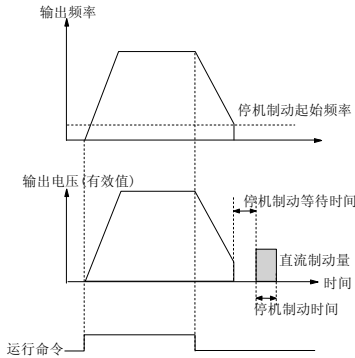
图 5-1-7 停机制动
