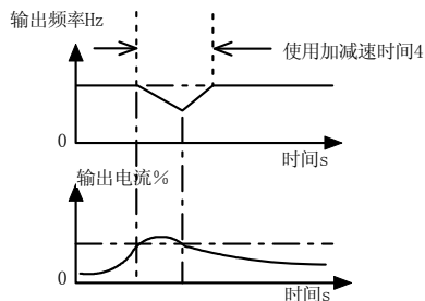
5-13-4 稳定运行过程
