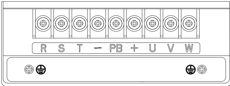
图 2-3 4KW~30KW 主回路端子接线
