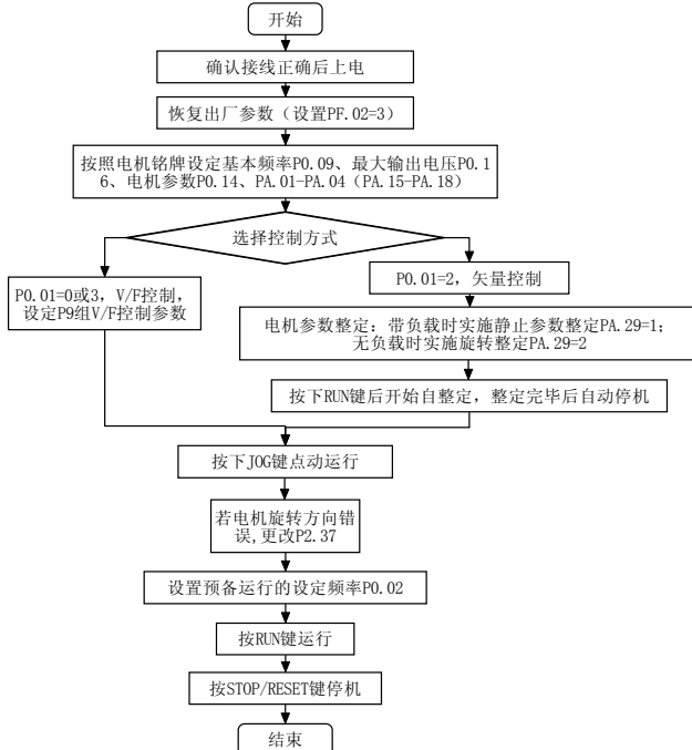
图 3-7 变频器首次试运行操作流程
