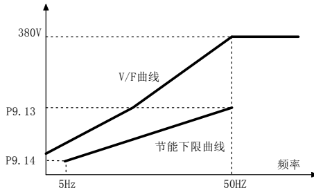
图 5-9-5 节能电压下限制
