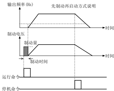
图 5-1-1 启动方式说明
