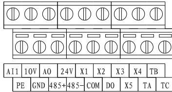
图 2-5 控制回路端子排布
