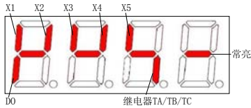
图 5-12-1 端子状态指示
