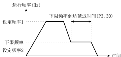
图 5-2-4 0频运行
