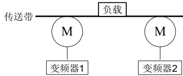
图 5-9-6 下垂控制电机特性
