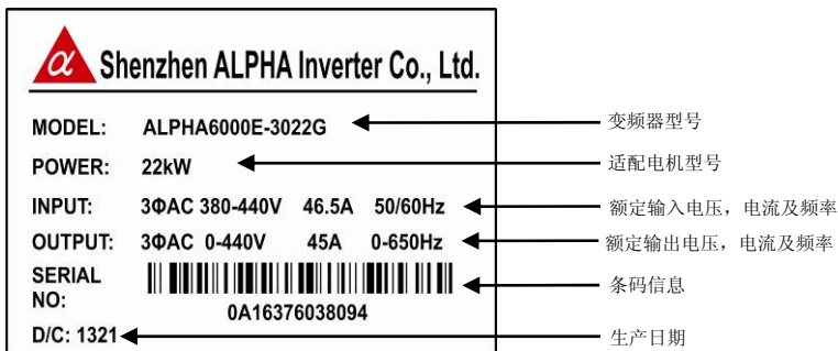
ALPHA6000E 系列变频器铭牌
