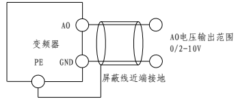
图 2-7 模拟输出端子配线图
