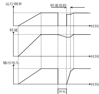
图 5-1-2 转速追踪
