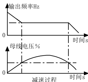
图 5-13-5 减速过程
