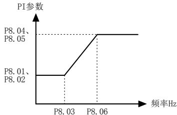
图 5-8-1 PI参数示意图
