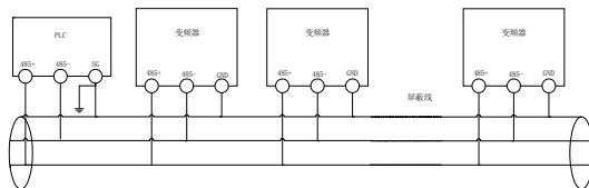
图 2-9 PLC与变频器多机通讯时推荐的接线图(变频器、电机全部良好接地)
