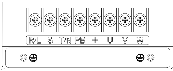
图 2-2 0.4kw~2.2kw 主回路端子接线
